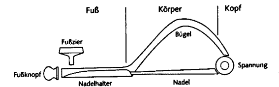
Bestandteile einer antiken Fibel am Beispiel einer Hallstattfibel.
